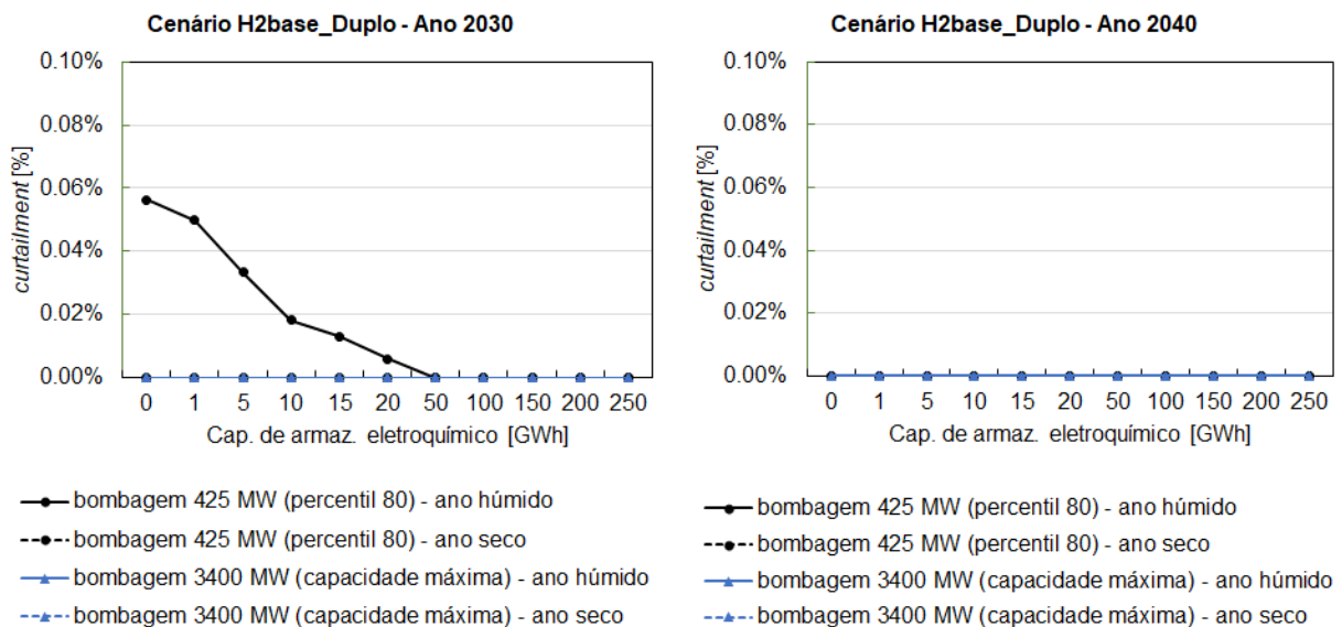
Figura 65 - “Curtailment” de energia em função da capacidade do armazenamento eletroquímico (baterias centralizadas) para duas capacidades de bombagem hidroelétrica disponível: 425 MW (equivalente ao percentil 80 de utilização) e 3400 MW (capacidade máxima) - Cenário H2base_Duplo.
