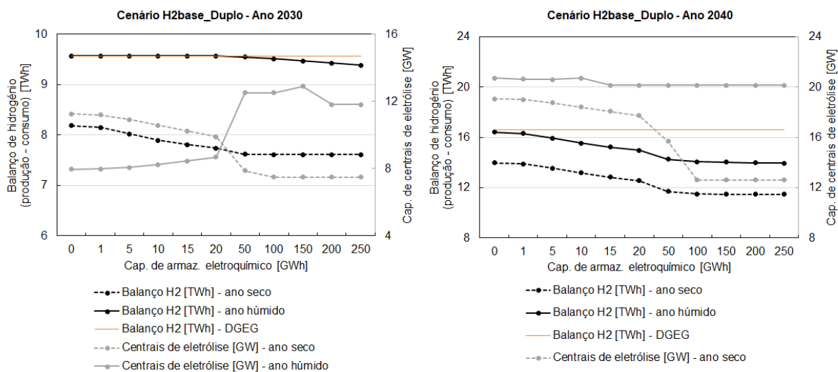
Figura 63 - Balanço de exportação-importação de hidrogénio e capacidade necessária de centrais de eletrólise em função da capacidade do armazenamento eletroquímico (células de combustível) - Cenário H2base_Duplo.
