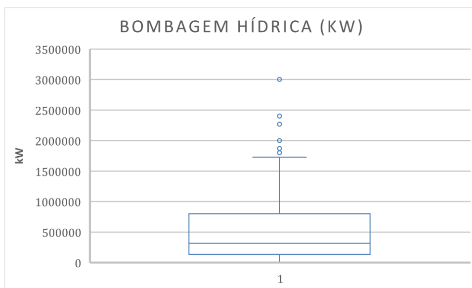
Figura 11 - Diagrama de extremos e quartis de bombagem hídrica no mundo. Fonte: 9 .
