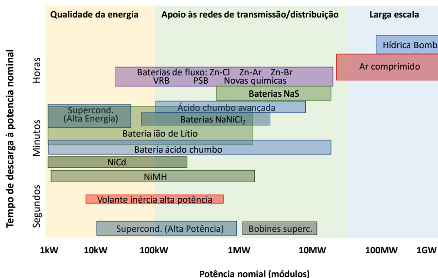
Figura 7 - Quadro conceptual de adequação de tecnologias de armazenamento de energia a três tipologias de aplicações: garantia de qualidade de energia, apoio às redes de transporte e distribuição e armazenamento de larga escala. Fonte: Adaptado de 78 .
