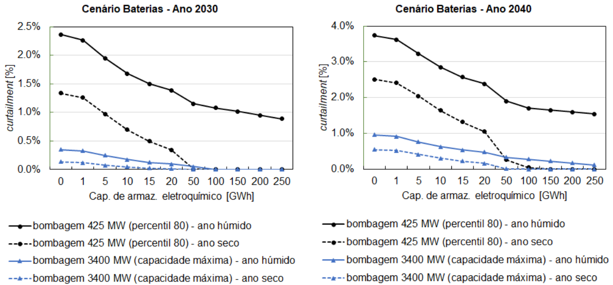
Figura 64 - “Curtailment” de energia em função da capacidade do armazenamento eletroquímico (baterias centralizadas) para duas capacidades de bombagem hidroelétrica disponível: 425 MW (equivalente ao percentil 80 de utilização) e 3 400 MW (capacidade máxima instalada) - Cenário Baterias
