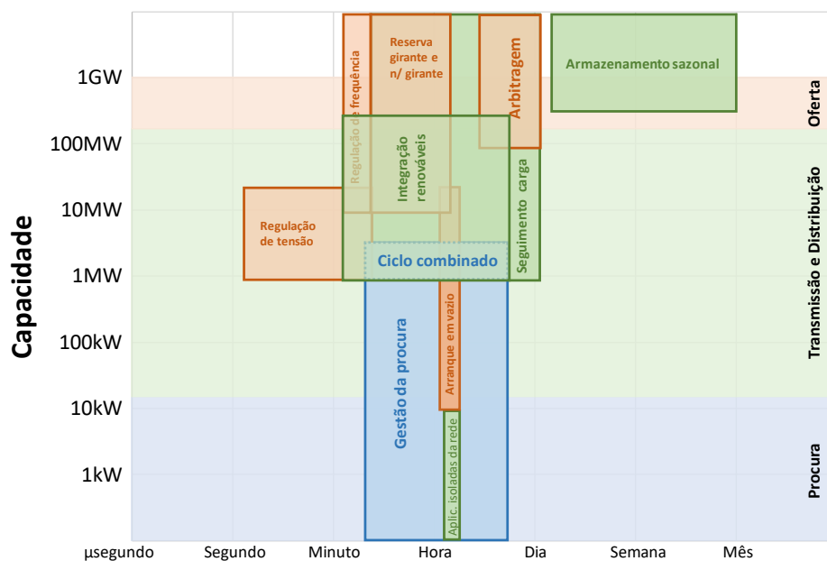
Figura 5 - Caracterização necessidades de potência e tempo de descarga dos diversos tipos de aplicações (laranja-aplicações elétricas; azul-aplicações térmicas; verde-aplicações térmicas ou elétricas). Fonte: Adaptado de 76 .
