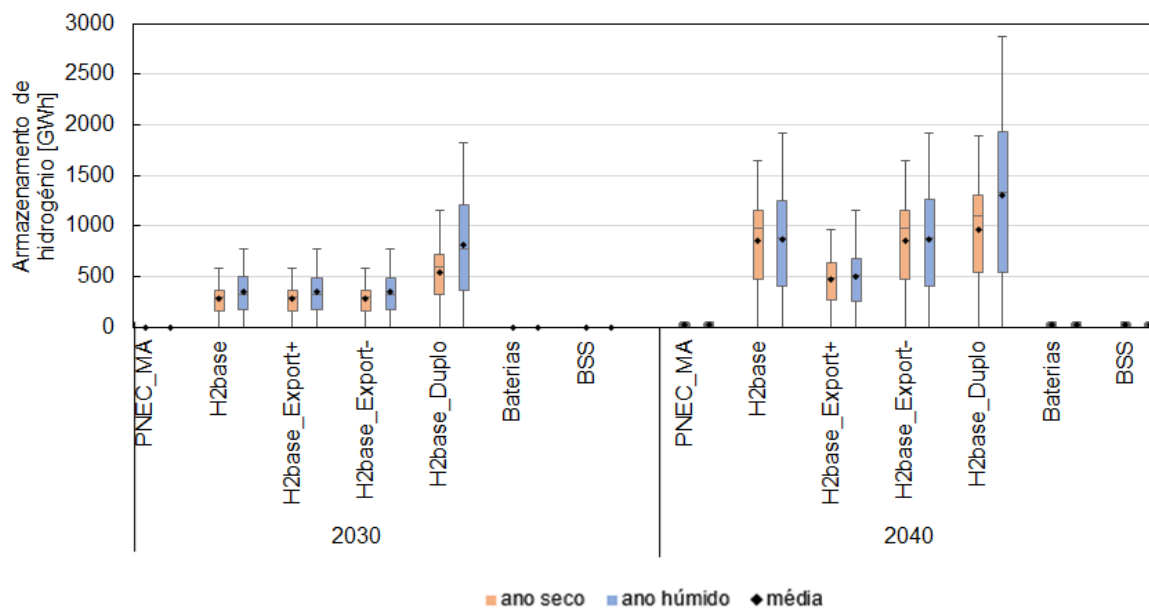
Figura 53 - Armazenamento de hidrogénio necessário ao longo do ano.
