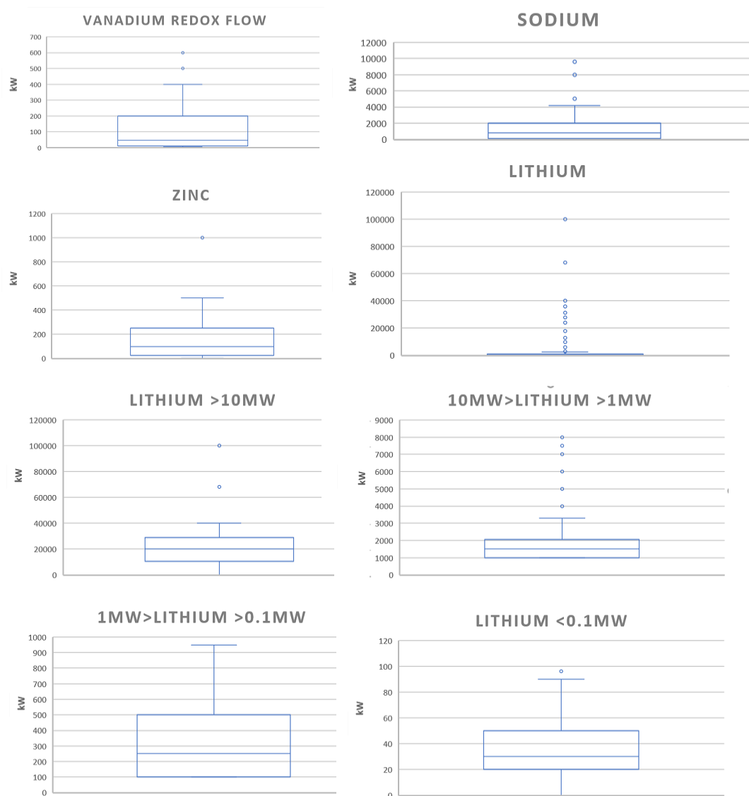
Figura 17 -Diagrama de extremos e quartis para diferentes tecnologias de baterias no mundo. Fonte: 9
