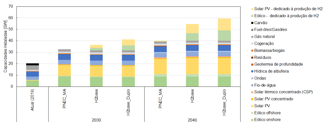
Figura 26 - Capacidades instaladas do parque eletroprodutor 90 .
