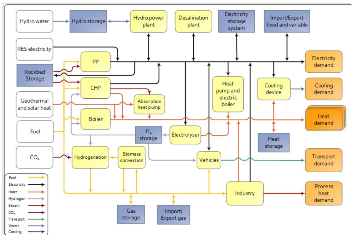
Figura 23 - Representação do sistema de referência no EnergyPLAN. A azul destaca-se as tecnologias disponíveis de armazenamento.
