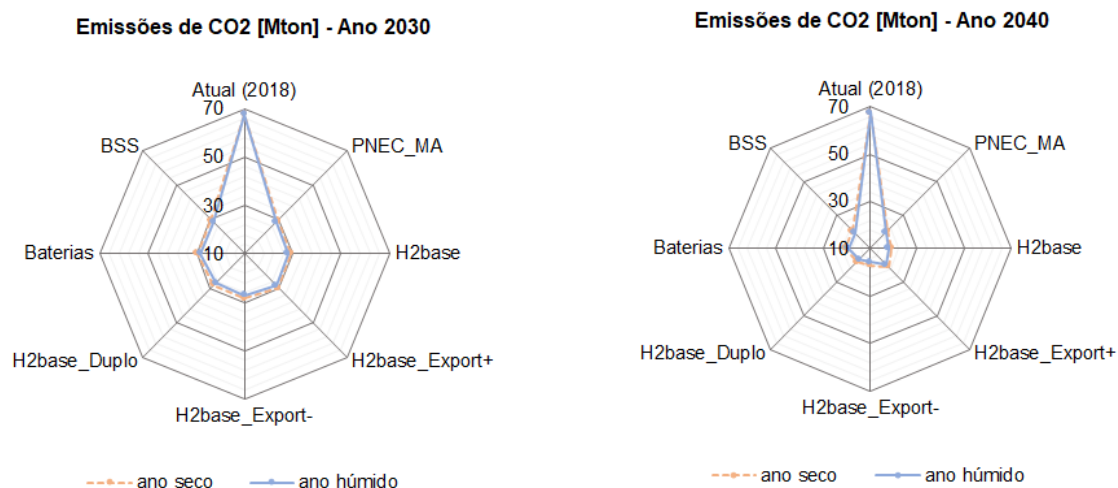
Figura 37 - Emissões de dióxido de carbono 107 .
