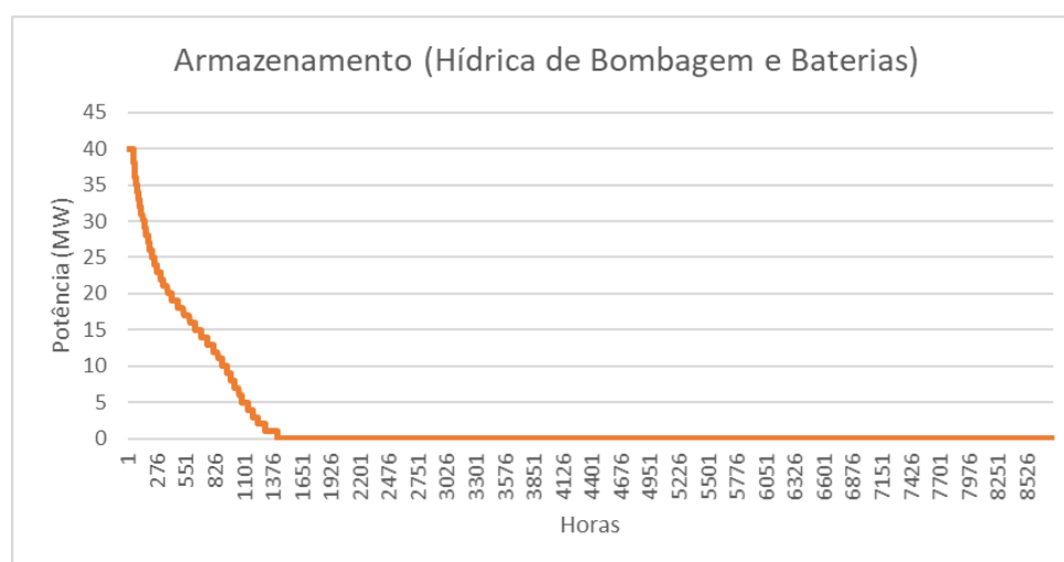
Figura 69 - Estimativa de Diagrama da duração de carga da hídrica de bombagem em 2030 (25 MW em bombagem hídrica e 15 MW em baterias), considerando potência mínima de central térmica de 22 MW e que a geração térmica representa no mínimo 20% da produção.
