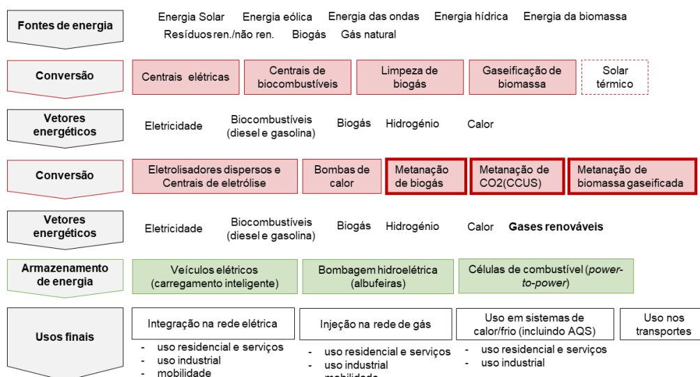
Figura 25 - Esquema representativo do sistema energético do cenário H2base para 2030 e 2040. Os retângulos destacados representam tecnologias de produção de gases renováveis para injeção na rede de gás não considerados na estrutura do sistema energético do cenário PNEC_MA.
