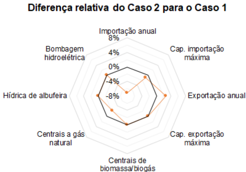
Figura 36 - Diferenças relativas de alguns dos principais indicadores de operação do sistema elétrico resultantes do Caso 2 (descentralizado) em relação ao Caso 1 (centralizado) apresentado a cor-de-laranja. A linha preta realça o valor 0% para todos os indicadores.
