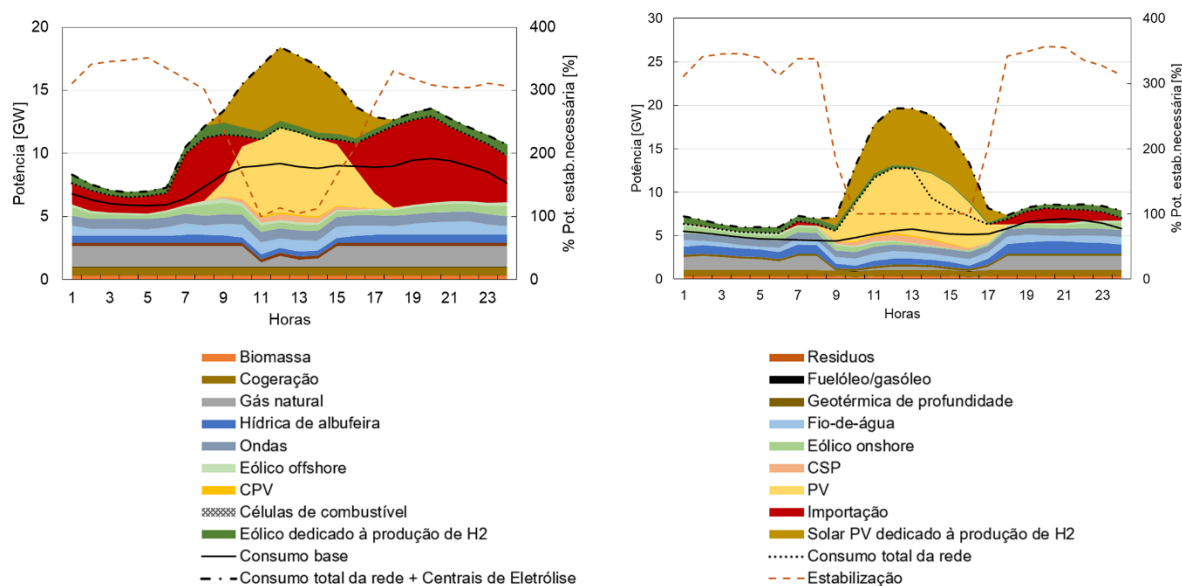
Figura 55 - Diagramas de carga para o dia com importação mais elevada no ano seco (à esquerda) e primeiro dia do ano no ano húmido (à direita) para o cenário H2base_Duplo em 2040. O consumo base corresponde ao consumo dos setores económicos exceto o transporte rodoviário. O consumo total da rede inclui o consumo base, os veículos elétricos, a bombagem hidroelétrica e as células de combustível.
