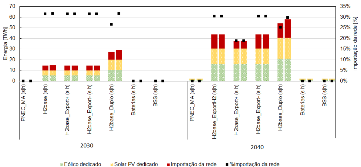
Figura 50 - Eletricidade para produção de hidrogénio (centrais dedicadas e importação do excedente da rede elétrica) e contribuição correspondente da importação da rede para essa mesma produção.
