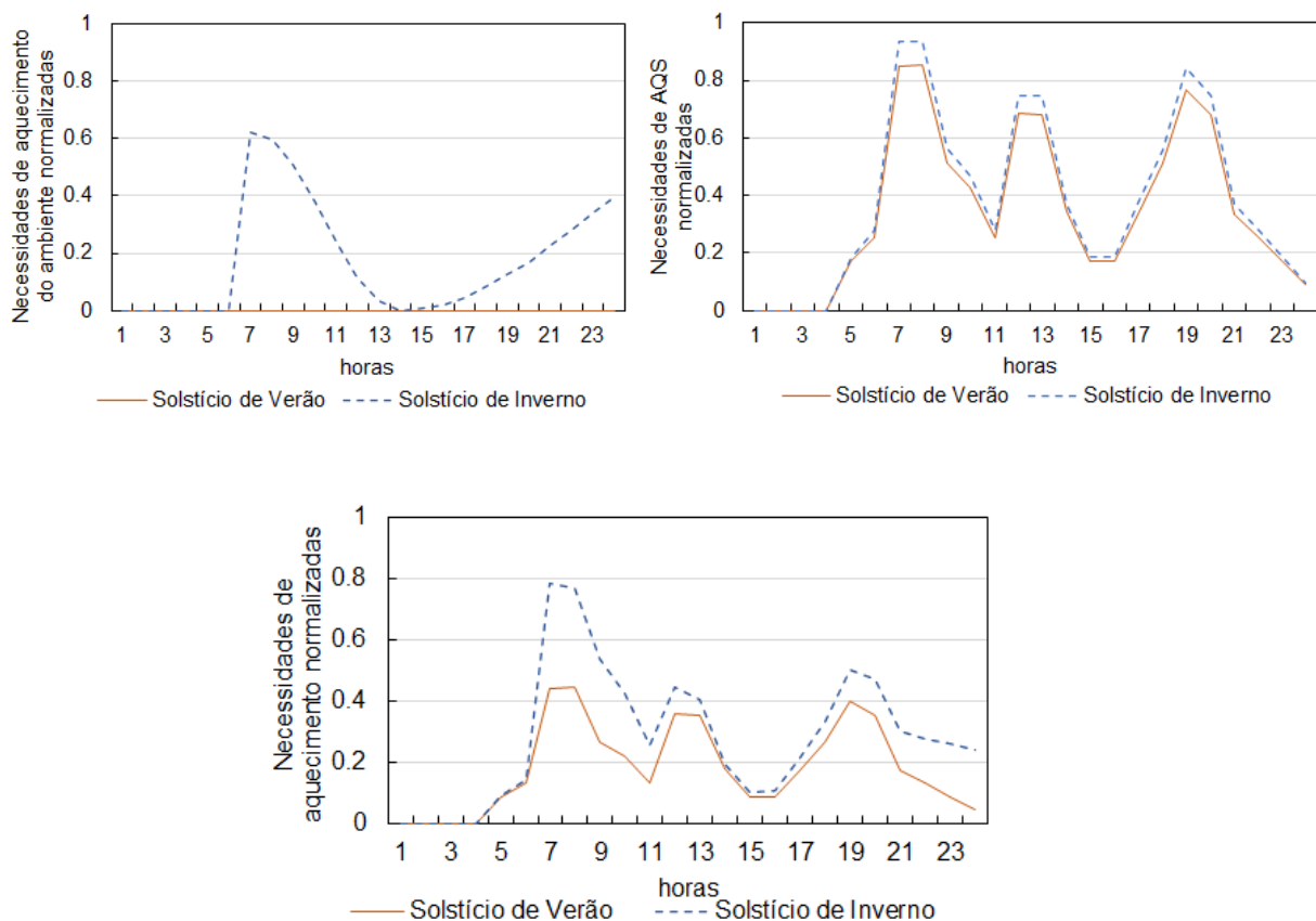
Figura 33 - Perfis normalizados das necessidades de aquecimento do ambiente (cima esquerda), de aquecimento de águas sanitárias (cima direita) e totais (baixo) para o dia do Solstício de Verão e de Inverno.
