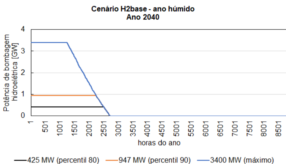
Figura 60 - Curva de duração da potência de bombagem hidroelétrica ao longo do ano para diferentes níveis de capacidade de bombagem disponível. Resultados para o ano húmido.
