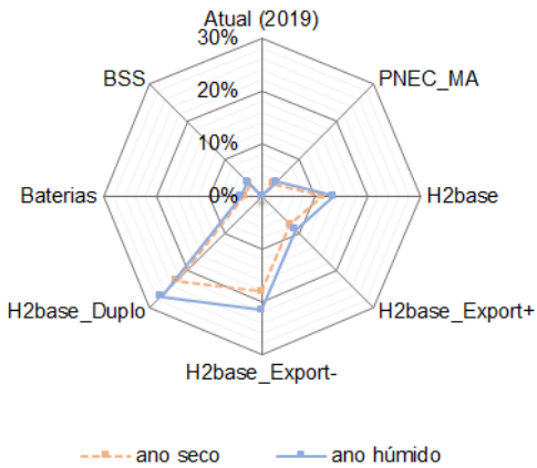
Figura 39 - Fração de energia renovável na rede de gás.
