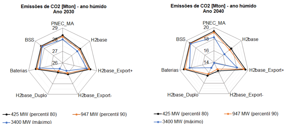
Figura 56 - Emissões de dióxido de carbono para diferentes níveis de capacidade de bombagem disponível. Resultados para o ano húmido.
