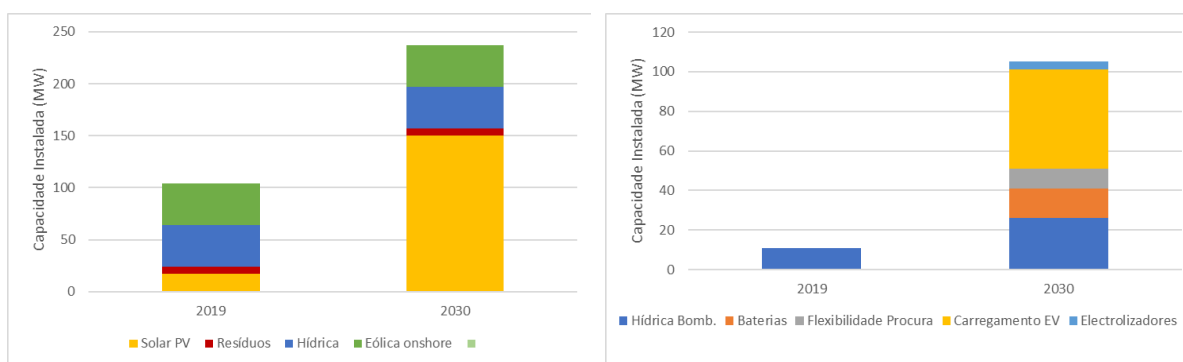
Figura 68- Capacidades instaladas de geração renovável (à esquerda) e armazenamento (à direita)
