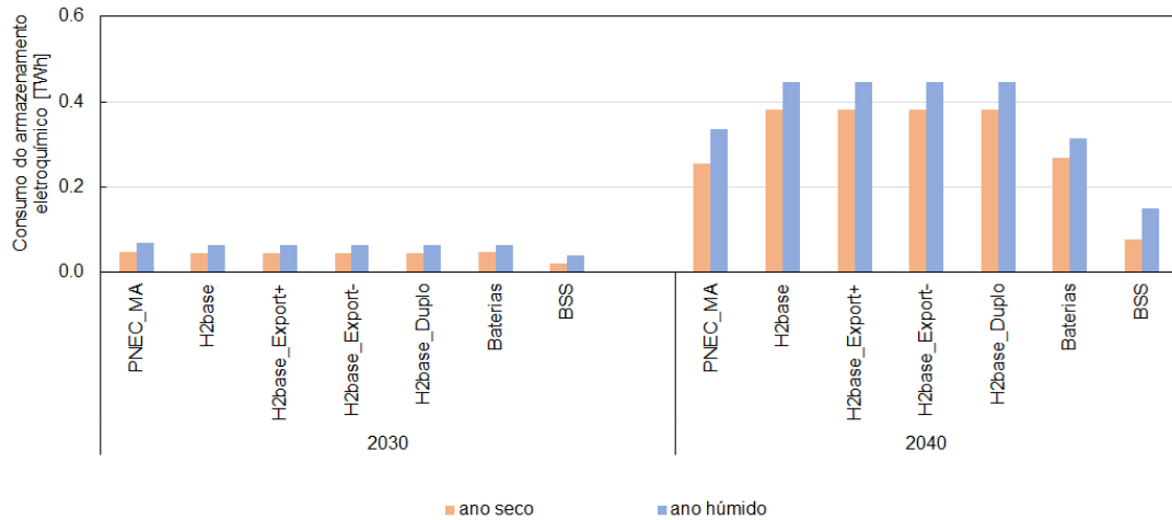
Figura 49 - Consumo anual de eletricidade para o armazenamento eletroquímico.
