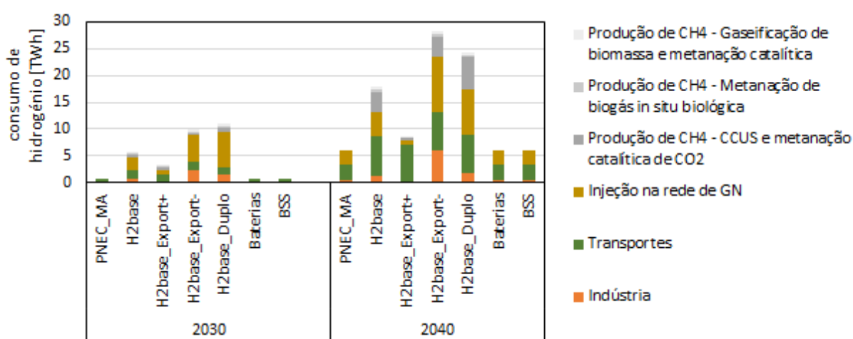
Figura 31 - Consumo de hidrogénio por tipo de utilização.
