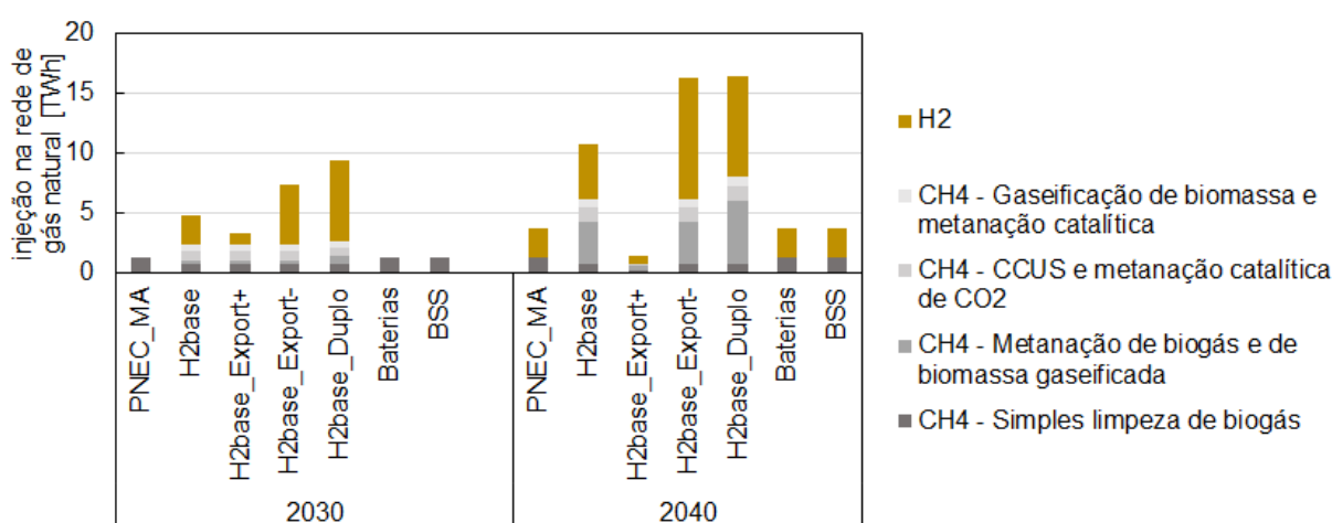
Figura 30 - Injeção de gases renováveis para na rede de gás.
