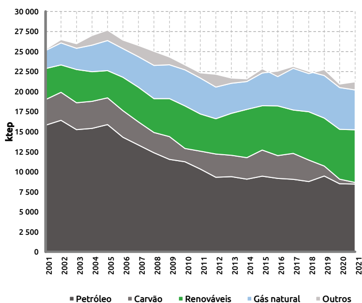
Fig. 26 Evolução do consumo total de energia primária
