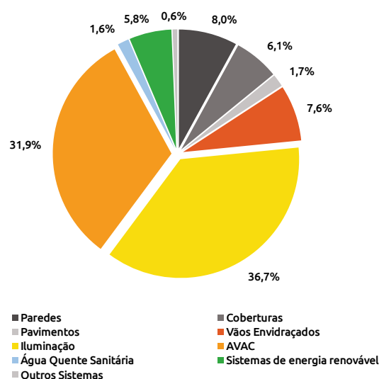
Fig. 120 Medidas de melhoria por âmbito de intervenção – comércio e serviços [2014-2022]
