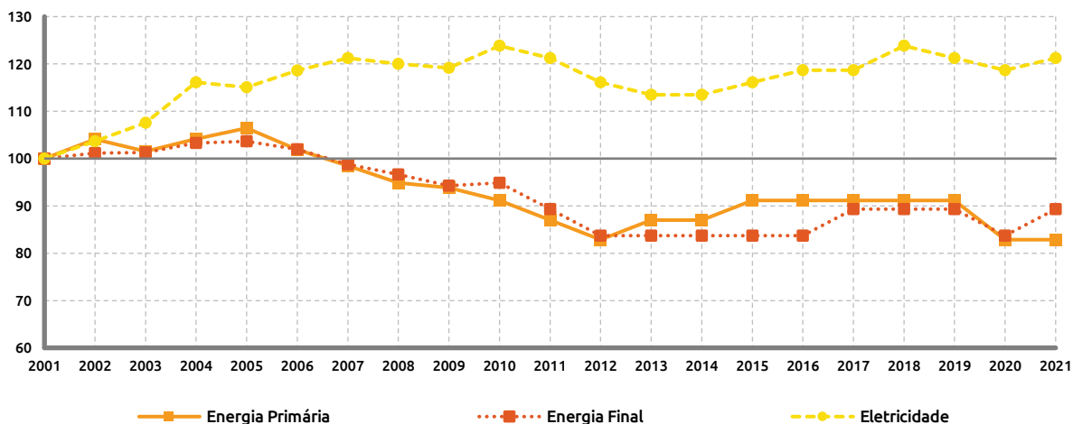
Fig. 10 Evolução do consumo de energia per capita (2001 = 100)
